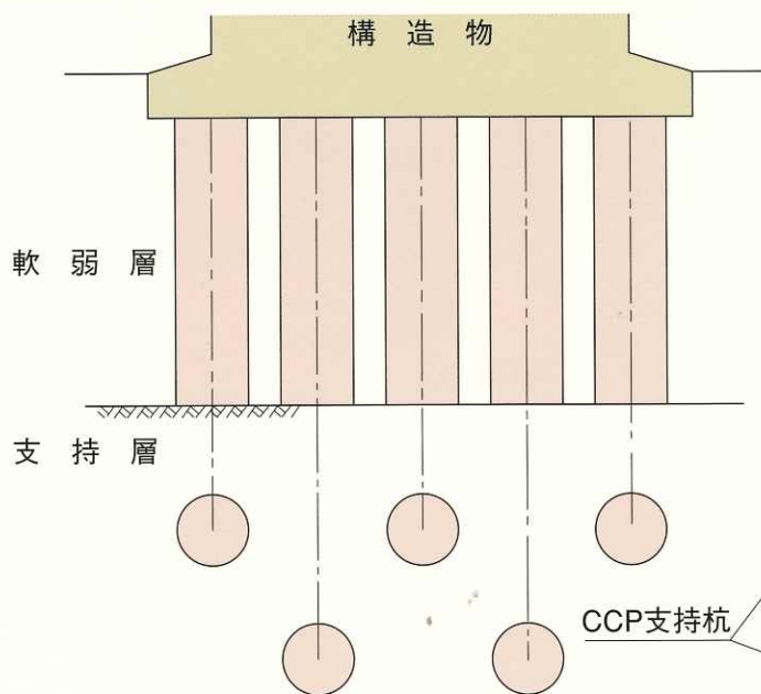
支持杭
