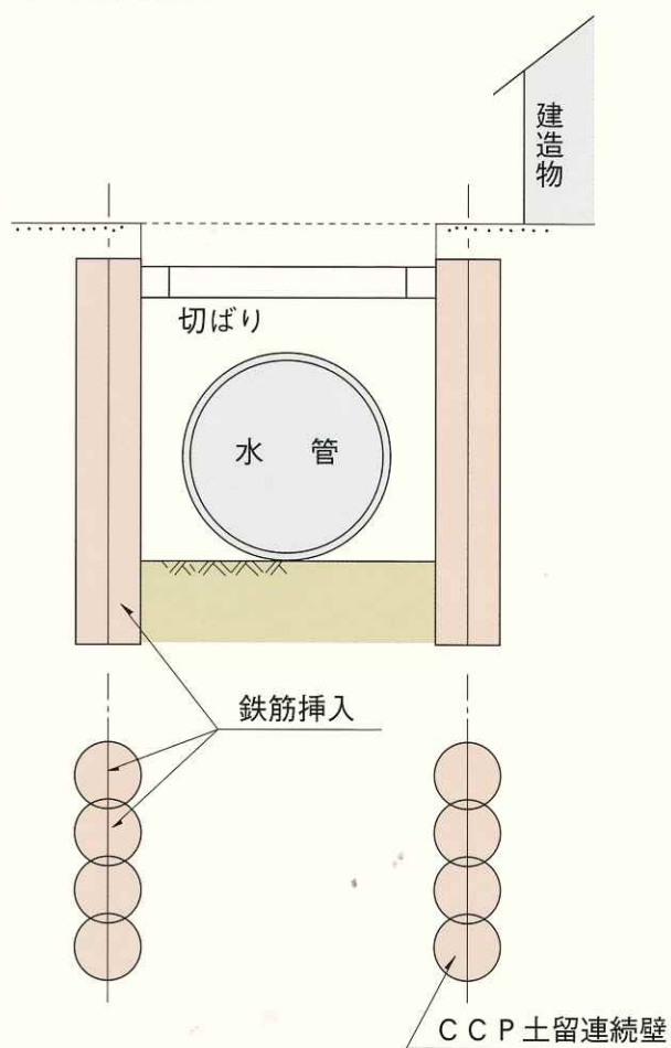
土留連続壁
