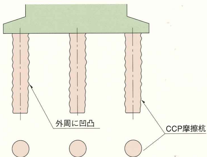
摩擦杭
